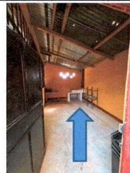
3.3 SUMINISTRO E INSTALACION DE TABLON DE CEMENTO EN COCINA 0.90 DE ALTO X 0.60 DE ANCHO X 8.5 MTS DE LARGO
