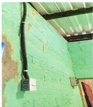
Foto 7: 3.4: INSTALACION DE APAGADORES SIMPLE
