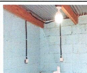
Foto 10 3.7: INSTALACION DE CAJAS RECTANGULARES
