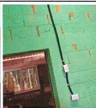
Foto 10 3.7: INSTALACION DE CAJAS RECTANGULARES
