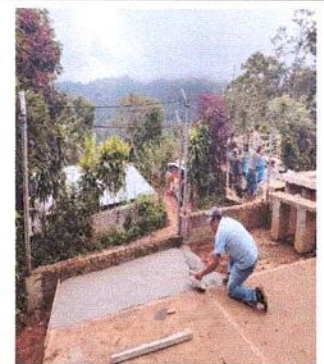
FOTO 4: 2.1 Sustitución de piso de tierra por entortado de cemento enfrente de aula lado derecho.
