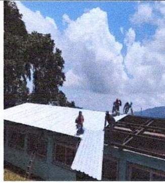
FOTO 1: 1.1 Sustitución de lámina, por lamina troquelada aluzinc calibre 26.
