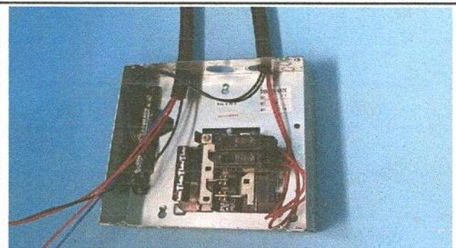
Foto 3: Instalación de cableado con caja de filpones
