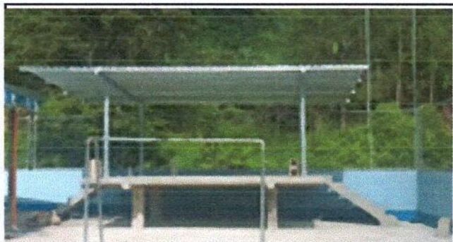
Foto 11: cambio de piso de madera por terraza de concreto a escenario. columna con zapata y corona para soporte de terraza del escenario
