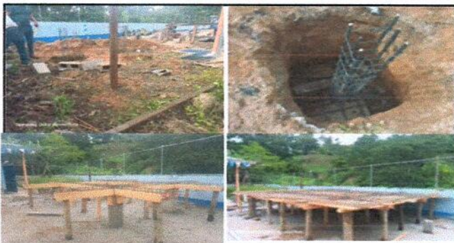
Foto 11: cambio de piso de madera por terraza de concreto a escenario.columna con zapata y corona para soporte de terraza del escenario
