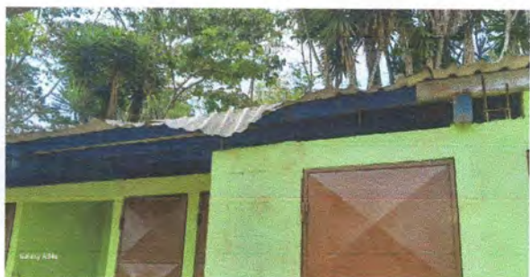
Foto 3: Matenimiento a estructura de soporte de metal, sustitución de lamina, por lamina troquelada aluzinc calibre 26, sustitución de soporte o pescante de metal para canal, sustitución de canal de metal y reparación de bajada de agua pluvial, tubo PVC 3".
