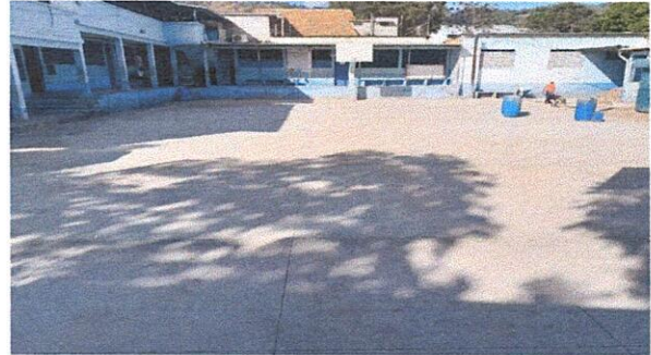
Foto 4: Finalización del fundición de 448 mts. Cuadrados de torta de cemento en cancha polideportiva: INEB JM. San Diego.
