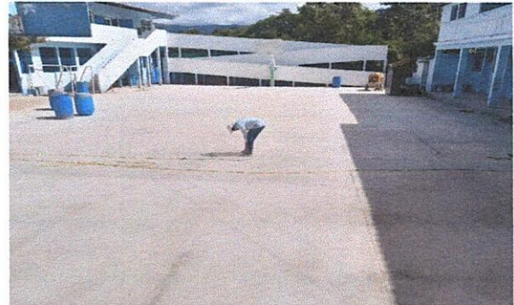
Foto 2: Finalización del fundición de 448 mts. Cuadrados de torta de cemento en cancha polideportiva: INEB JM. San Diego.
