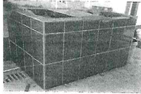
Foto 2: SUSTITUCIÓN DE PILA DE PLÁSTICO POR PILA DE BLOCK Y CONCRET.O E INSTALACIÓN DE AZULEJO EN COCINA
