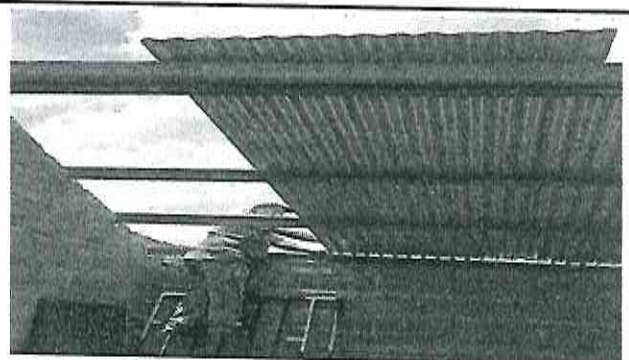
Foto 6: Sustitución de lámina ondulada por lámina troquelada calibre 26 aluzinc
