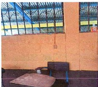
Foto 17: Aula 5: Retiro de cable electrico existente, colocación de cable calibre 10, Flaponeras, Bombillas de 40 amperios, Instalación de apagadores dobles.
