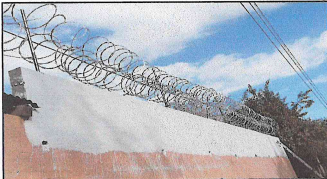
LEVANTAMIENTO DE BLOCK SOBRE MURO PERIMETRAL EXISTENTE 4 HILADAS Y SUMINISTRO E INSTALACION DE RAZOR GALVANIZADO, ESTO MITIGARA QUE LADRONES ENTREN AL ESTABLECIMIENTO A ROBAR, LA EDIFICACION SI PERMITE LEVANTAR LAS 4 HILADAS DE BLOCK
