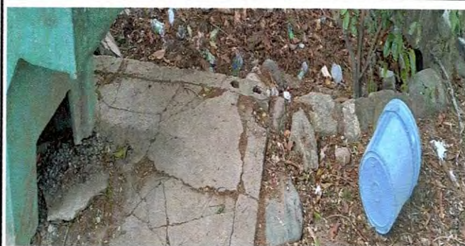
Foto 10: Aquí se observa los daños que posee la losa de patio que se desea reemplazar
