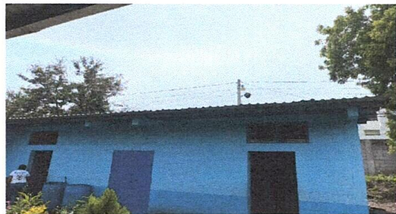
foto 18: instalación de canal de metal mas pescantes e instalación de bajada de agua pluvial de tubo PVC 4"
