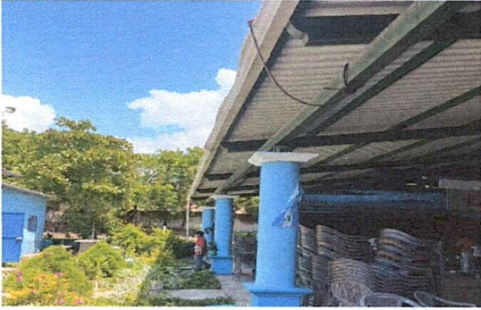
foto 13: sustitución de canal pvc por canal de metal mas pescantes y sustitución de bajada de agua pluvial.
