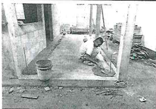
Foto 12: Suministro e instalación de piso de torta de concreto
