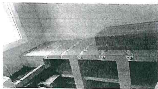
Foto 9: Sustitución de estufa rural completa (Incluye polletón. Plancha metálica y chimenea)
