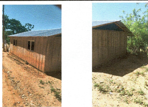
Foto 2: Sustitución de estructura de madera en paredes
