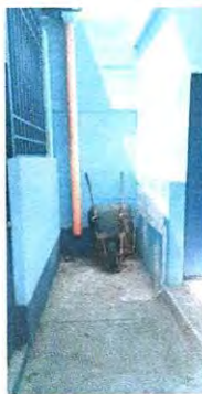
Instalación de lavador de concreto con azulejo y su respectivo chorro.
