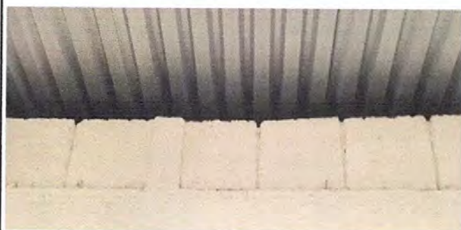
Foto 6: SELLADO DE GRIETAS CON CEMENTO CICLOPIO Y TAQUIQUES DE 7X19X39 ENTRE VIGA DE CORONA Y TECHO
