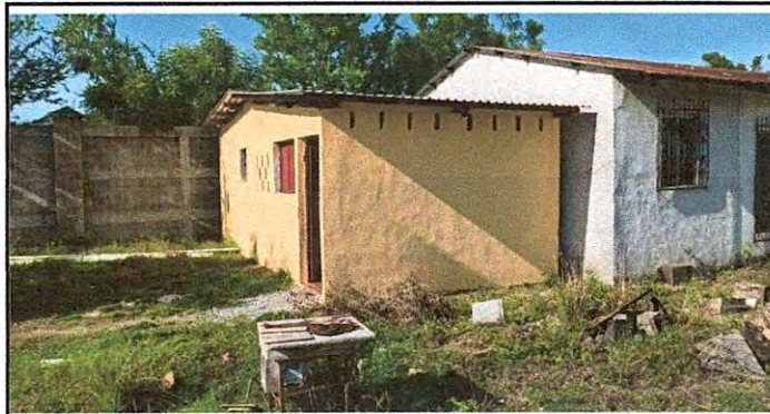
Foto 2: Levantado de Muros, Repellos y Cernidos (Se subirán 3 Hiladas de Block) en Cocina
