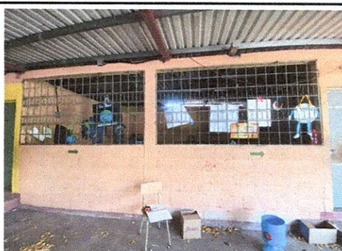
Foto 4: Reparación de muro de block aplicando cernido ( incluye cepillar la pared para eliminar la pintura existente) en las aula 2 y 3
