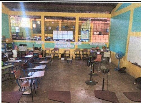
Foto 11: Sustitución de interruptores simples, Sustitución de tomacorrientes dobles, Instalación de ventilador de techo, pintura en muro interior en aula 5
