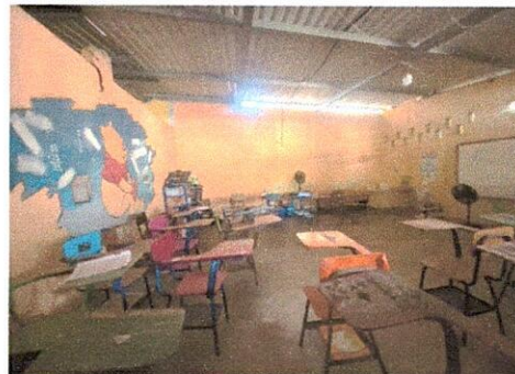
Foto 6: Sustitución de interruptores , Sustitución de tomacorrientes , pintura muros interiores, instalación de ventilador, reparación de Muro pegando 3 hiladas de block para elevar el techo con repello y cernido en
