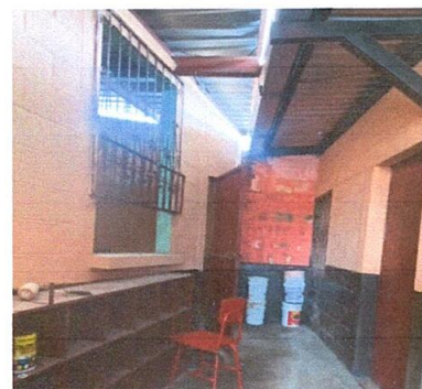
Foto 4: construcción de pila de cemento de un lavadero con azulejo en la parte exterior de 1.50x1.20 mts en la cocina, instalación de tubería para agua potable, instalación de tubería para aguas grises
