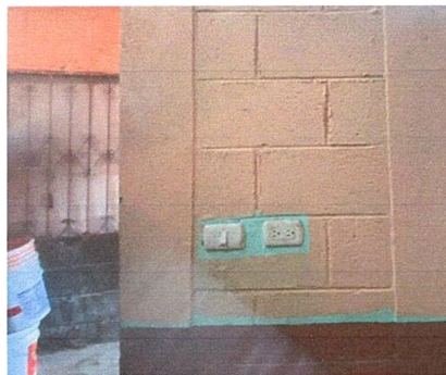
Foto 2: Sustitución de tomacorrientes dobles, sustitución de interruptor simple por interruptor doble en la cocina
