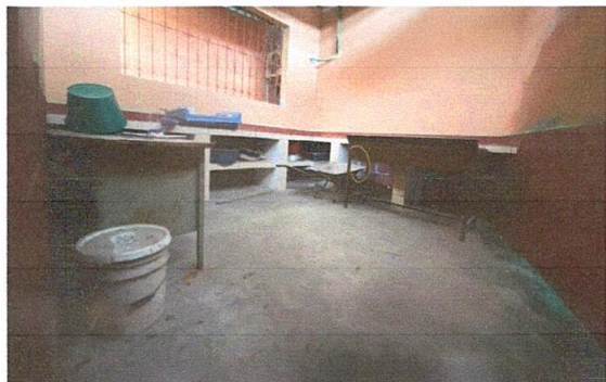
Foto 1: Sustitución de piso de torta de concreto por piso cerámico con zócalo, reparación del piso de torta de concreto para nivelar la base, instalación de azulejo en la parte superior del gabinete bajo en la cocina
