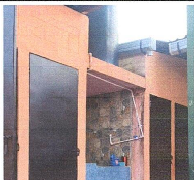
Foto 15: Sustituir tubería de pvc de agua potable del rotoplas para la pila por tubería de pvc nueva, sustitución de llave de paso de pvc por llave de paso de metal en el rotoplas del servicio sanitario
