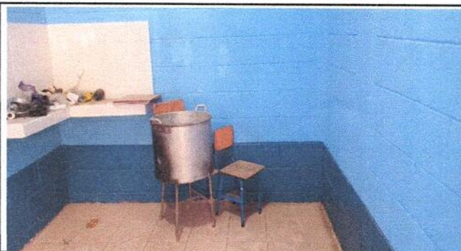
Foto 5: Instalación de Mueble de Concreto y Azulejo en Cocina
