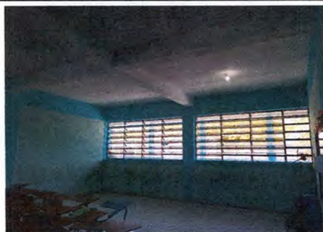
Foto 11: Instalacion de pared de material tabla yeso para división del aula
