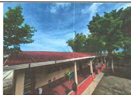
Foto 6: Sustrucción de lamina por lamina troquelada prepintada calibre 26 en aulas 11 y 12
