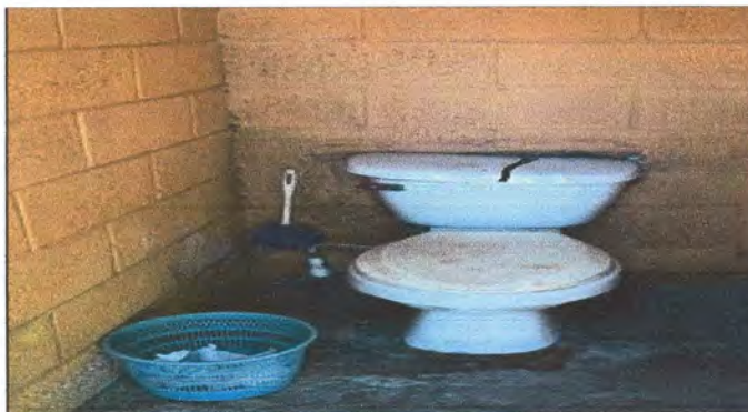
Numeral 2.1 Sustitucion de Inodoros en mal estado, llave de paso, tubo de abastecimiento e inodoro y tanque completo con accesorios
