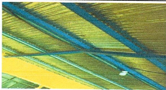
Foto 7: SUSTITUCIÓN DE LÁMINA, POR LÁMINA TROQUELADA ALUZINC CALIBRE 26 Y MANTENIMIENTO A ESTRUCTURA DE SOPORTE DE METAL
