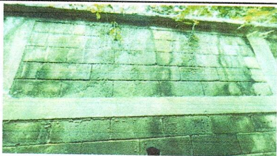
Foto 9: SUSTITUCIÓN DE BLOCK DAÑADO EN MURO PERIMETRAL Y REPLLO / EL MURO YA SE ENCUENTRA MUY DEBILITADO
