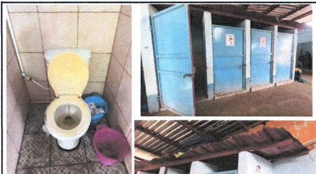
Foto 8: SUMINISTRO E INSTALACIÓN DE PUERTA DE METAL EN BAÑOS (MATERIAL Y MANO DE OBRA) (MEDIDAS= 0.88 ANCHO * 2.00 ALTO) /SUSTITUCIÓN DE LÁMINA POR LÁMINA TROQUELADA CALIBRE 26 /SUSTITUCIÓN DE 2 INHODOROS
