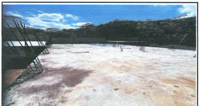
Foto 4: Ponerle Pañuelos a una parte de la terraza pegada de lado del escenario ya que sufre de humedad
