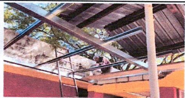
Foto3: Después de haber hecho la instalación de estructura de tubos y costaneras, se procedió a nivelar la vigas de agua pluvial con block, cemento y arena en el módulo del pasillo que queda enfrente del Salón de Conferencia
