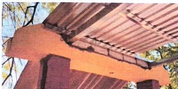
Foto3: Después de haber hecho la instalación de estructura de tubos y costaneras, se procedió a nivelar la vigas de agua pluvial con block, cemento y arena en el módulo del pasillo que conduce hacia el Área de
