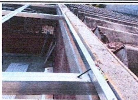
Foto 2: Se reconstruyó los laterales de los canales de agua pluvial en un módulo del Salón de Clases de área de carpintería.
