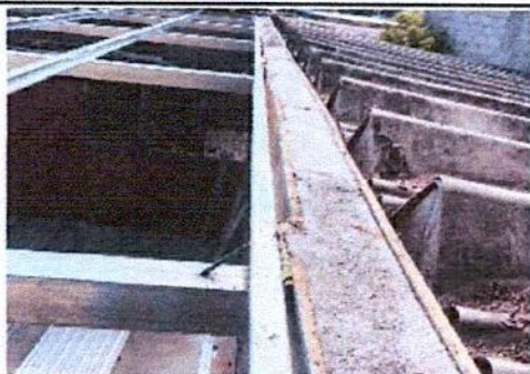
Foto 1: Después de haber hecho la demolición del techo y de haber instalado los tubos y costaneras, se procedió a restaurar los laterales de los canales de agua pluvial en un módulo del Salón de Clases de área de carpintería.
