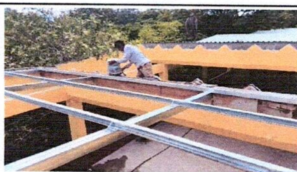
Foto 4: continuando con la instalación de los tubos y costaneras, se revisa que todo este bien antes de la instalación de las láminas
