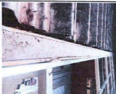
Foto 3: La reconstrucción los laterales de dichos canales, se hizo con cemento y arena, rellenando las ondulaciones donde se encontraba la duralita en un módulo del Salón de Clases de área de carpintería.
