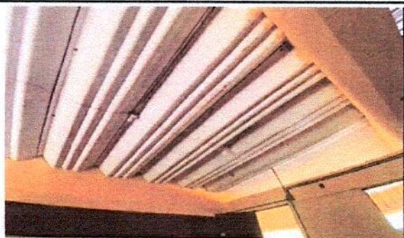
Foto 1: Aquí se esta inspeccionando la modalidad de botar el techo de un módulo del salón de clases y pasillo, de Segundo Grado E
