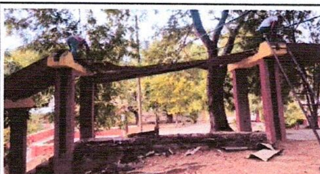
Foto 4: Seguimiento botar la lámina duralita del techo de un módulo que conduce al área de Segundo Grado Básico.
