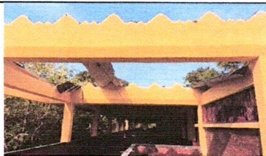
Foto 6: Seguimiento de demolición de techo en los módulos del Salón de clases y pasillo Segundo Grado Sección F.
