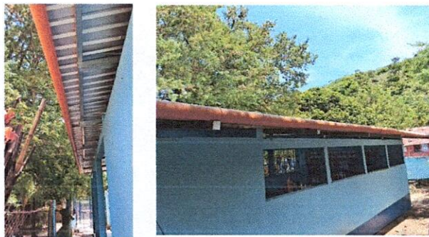
Foto 10: Sustitución de canales de pvc por canales de lámina aluzinc.
