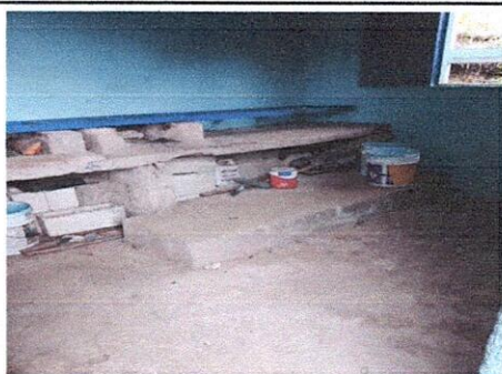
Foto 11 : Instalación de Mueble de Concreto, Drenaje de Aguas Servidas y Agua Potable en Cocina
