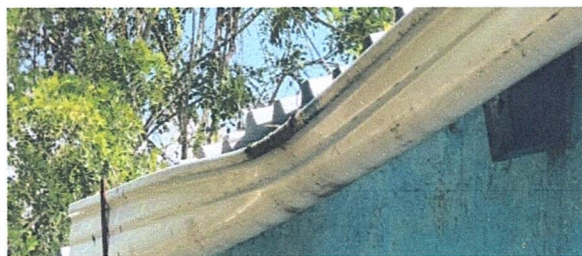
Foto 6: SUSTITUCIÓN DE CANAL PVC A CANAL DE METAL, SE REALIZARÁ EL CAMBIO PORQUE EL ACTUAC CANAL SE ENCUENTRA DETERIORADO AL SER DE PVC ES MENOS RESISTENTE, POR TAL MOTIVO SE CAMBIARÁ A CANAL DE METAL YA QUE CUENTA CON MAYOR DURABILIDAD Y RESISTENCIA.
