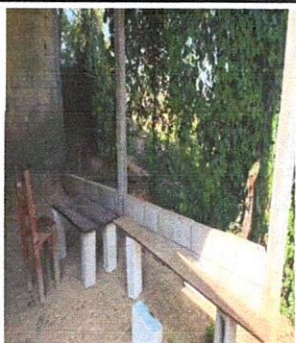
Foto 7: REPARACIÓN DE MURO PERIMETRAL DE BLOCK CON TUBO HG Y MALLA GALVANIZADA, SOLERAS INTERMEDIAS Y COLUMNAS
