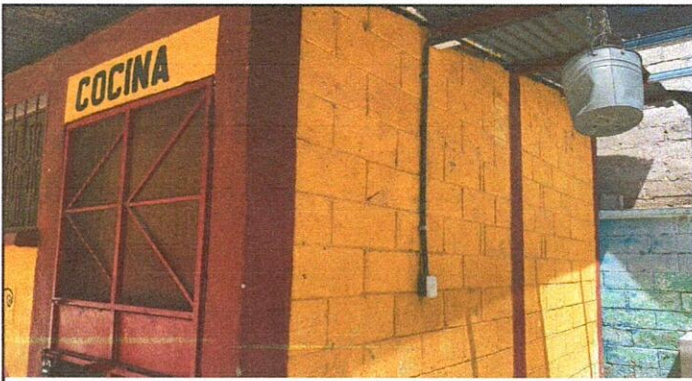
Foto 3: Pared lateral de cocina, donde se abrirá un espacio para ventana con la finalidad de darle mayor ventilación a la cocina escolar.
