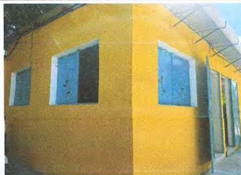
Foto 10: Modificación de ventanas abatibles a tipo caceta de 1*1.5, Suministro e instalación de Tapasol de 4.35*1.3 para ventanas donde pega el sol Y Puerta con tipo cedazo (marco metalico y cedazo fino) 1.4*2 4.6
