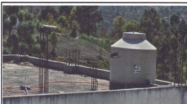
Foto 4: Mejoramiento de sistema de agua, compra de tinaco de 2500 ml
