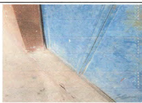
Foto 4: Reparación de media puerta de metal, por abertura con el marco en el lado izquierdo abajo.
