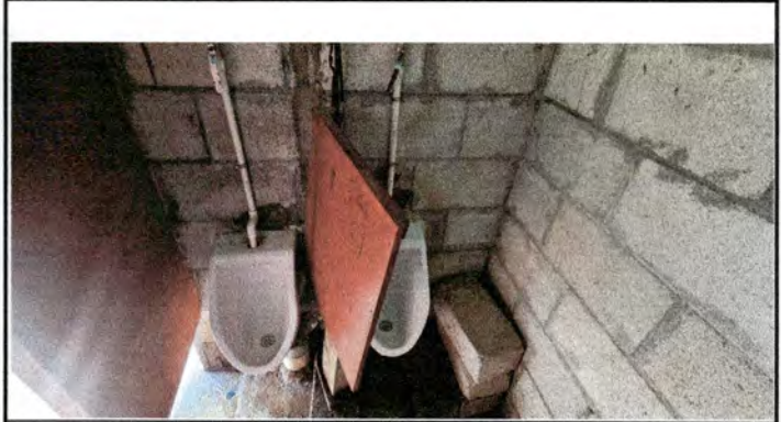
Foto 2: Sustitución de inodoros y migitorios de los baños, sustitución de piso de torta de cemento por piso ceramico.
