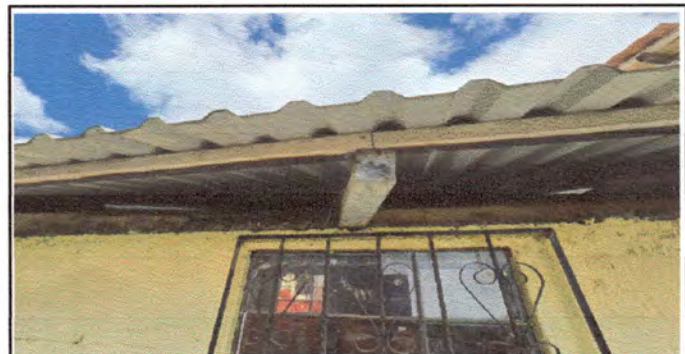
Foto 6: Parte de atrás de aulas, techo portante de madera en malas condiciones
