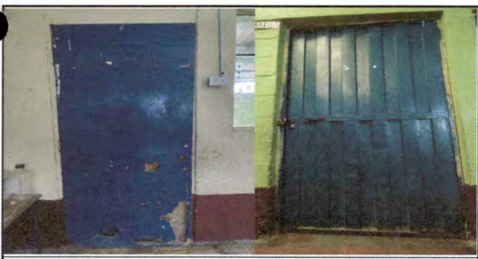
Foto 11: Fabricación e instalación de puerta metálica tipo abatible, diseño estructural liso, con tubo base de 1 pulgada y lámina lisa de 1mm, de 100cm de ancho y 210cm de alto, protegido con anticorrosivo color azul.
