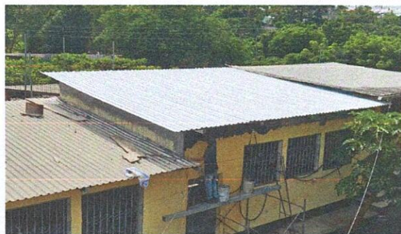
Foto 1: Cambio de lámina, tipo troquelada calibre 26
