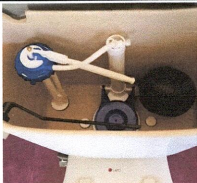
FOTO 5: Sustitución de accesorios de inodoros.
