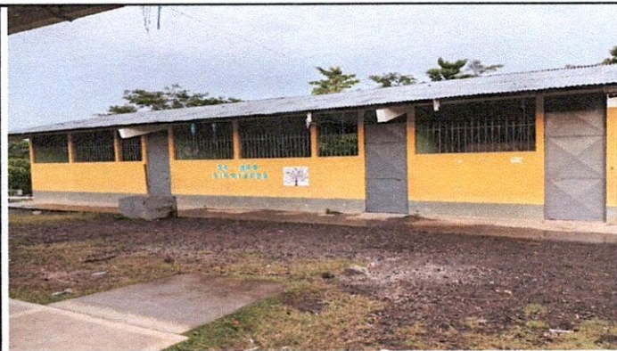
FOTO 3: Suministro de balcón de hierro 1/2", Mantenimiento de puertas de metal de 1.00 x 2.00 (cepillado, lijado y aplicación de pintura).
