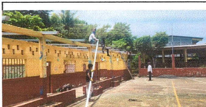
FOTO 4: SUSTITUCIÓN DE LÁMINAS, POR LAMINAS TROQUELADAS ALUZINC CALIBRE 26, SUMINISTRO DE ESTRUCTURA PORTANTE DE METAL.
