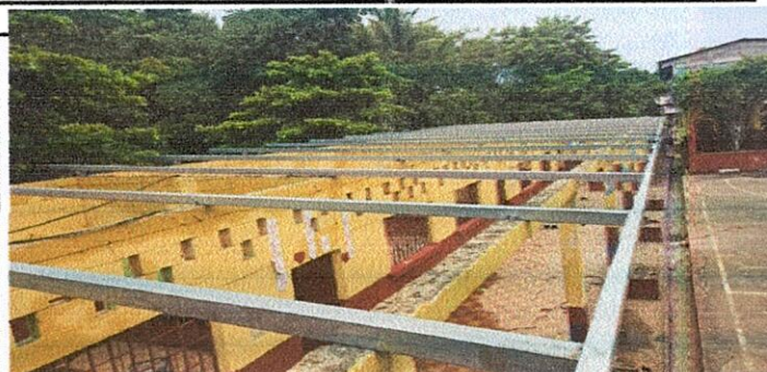
FOTO 5: SUSTITUCION DE LAMINAS TROQUELADAS ALUZINC CALIBRE 26. SUMINISTO DE ESTRUCTURA PORTANTE DE METAL
