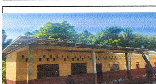
FOTO 6: SUSTITUCIÓN DE LAMINAS, POR LAMINAS TROQUELADAS ALUZINC CALIBRE 26, SUMINISTRO DE ESTRUCTURA PORTANTE DE METAL.
