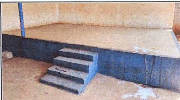
Foto 9: Sustitución de piso de torta de concreto por piso cerámico antideslizante
