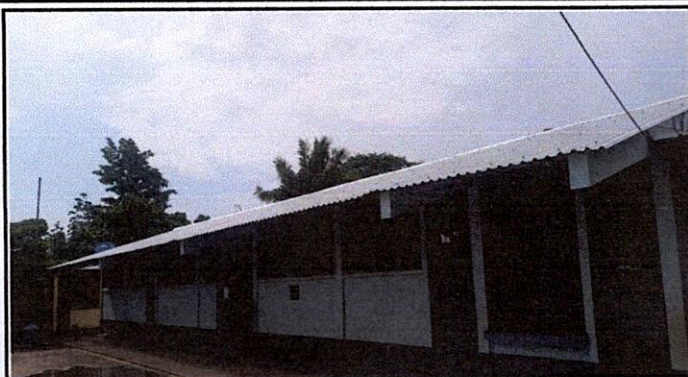
CAMBIO DE TECHO POR LAMINA TROQUELADA CALIBRE 26
