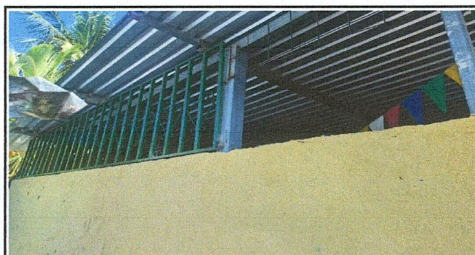
Foto 4: Sustitución de balcón de metal por marco 1"x 1" reforzado con hierro 3/8"
