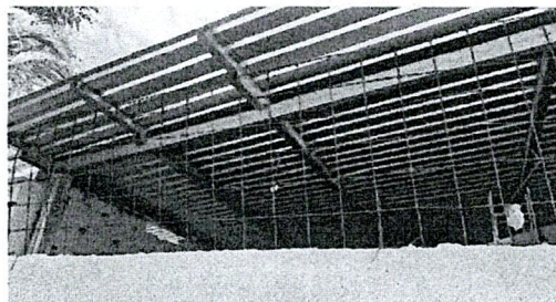
Foto 4: Sustrucción de balcón de metal por balcón de metal marco 1" x 1" reforzado con hierro 3/8"
