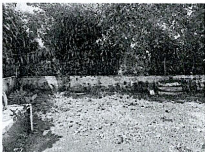
Foto 3: Suministro de block para circulación de muro perimetral (Incluye columnas de 0.15 x 0.15 x 1.00 mt con hierro Ø 1/2" est. 1/4 + solera de 0.20 x 0.15 con hierro Ø 3/8" est. 1/4")
