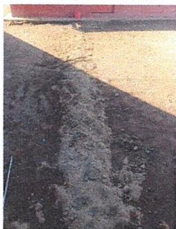
Foto 1: Sustrucción de tubería por tubería PVC Ø 4" (incluye zanqueo, compactación, colocación de tubería y relleno)
