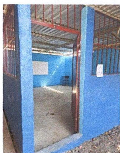
Foto 5: Sustrucción de costanera de madera por costanera metálica 2 x 3, Sustrucción de lámina por lámina troquelada cal. 26
